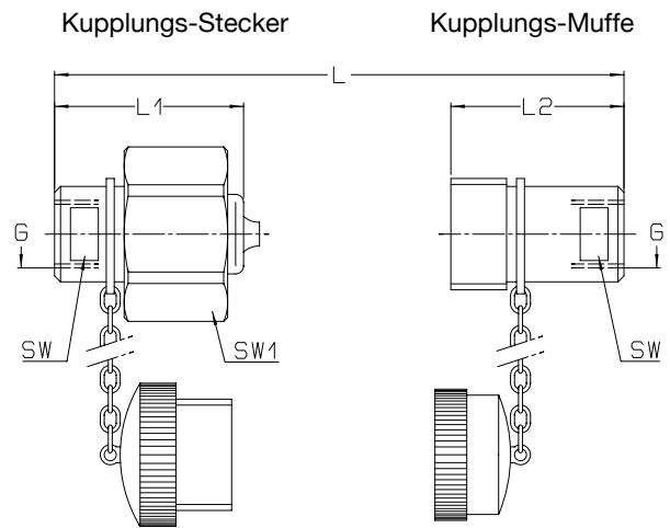
L = Gesamtlänge gekuppelt
